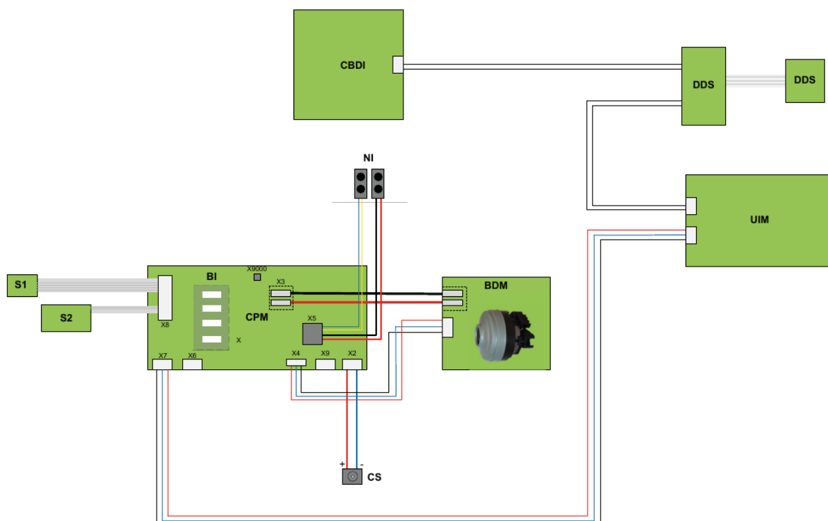
1. ábra: Csatlakozási rajz
